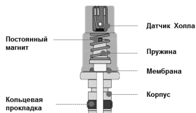
Принципиальная схема
