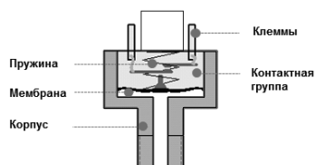
Принципиальная схема
